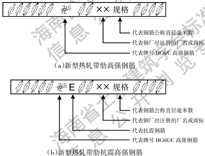
图 A.5.3 钢筋标志图例
